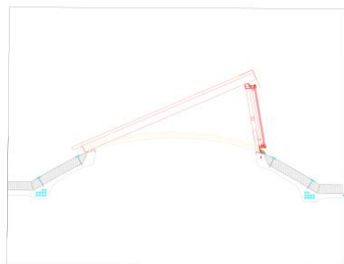
particolare 1:20
